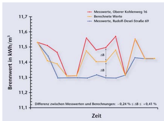
Vergleich gemessener und berechneter Brennwerte an zwei Kontrollpunkten
